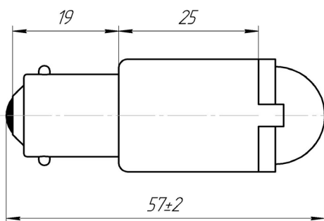
Габаритный чертеж
